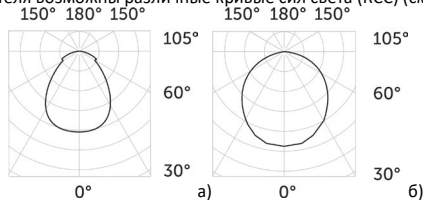
Рисунок 3: а) Микропризма 90°, б) Опал поликарбонат (120°).
