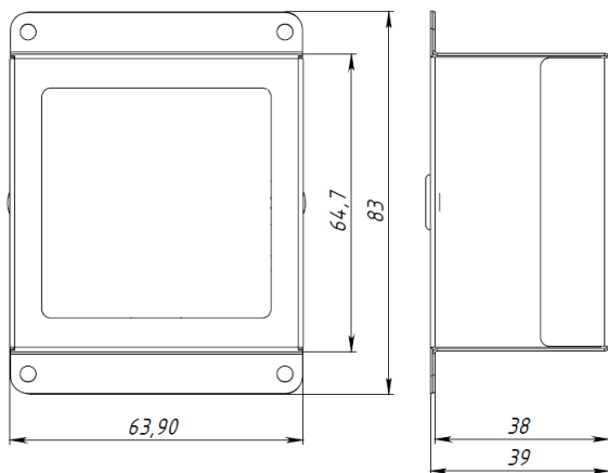
Рисунок 1 — Габаритные размеры светодиодного модуля Geniled Griliato Tetrис.
